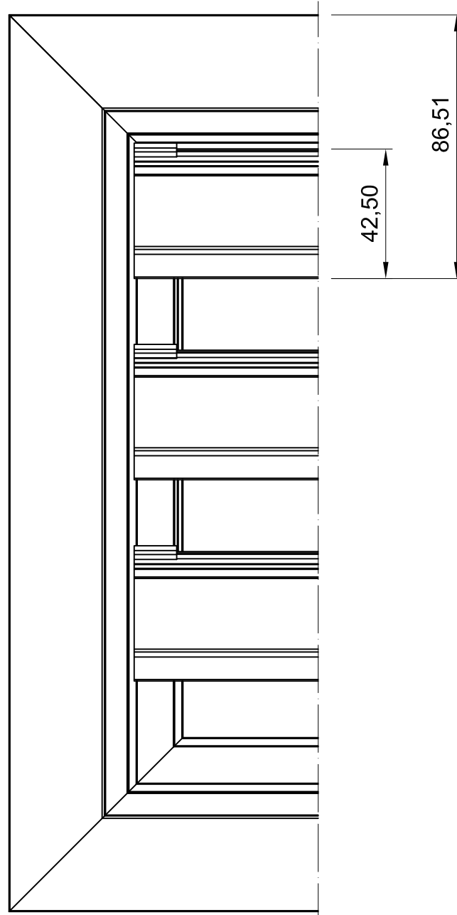
Vorderansicht
