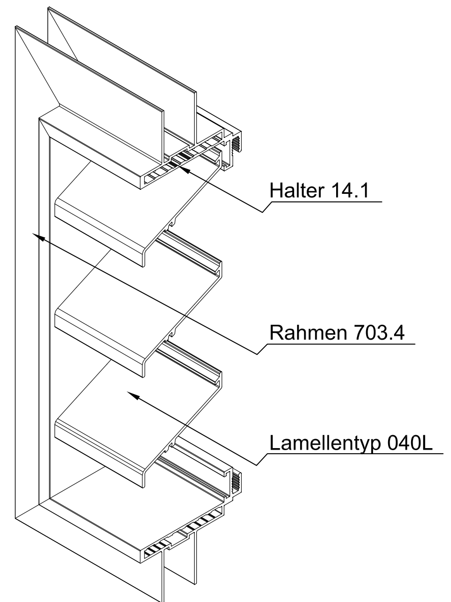
ISO-Ansicht
